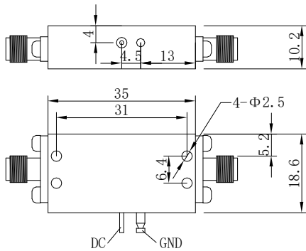
XB-02A UNIT: mm
