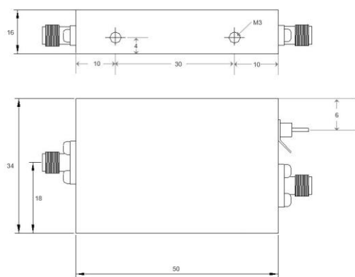
XB-06C UNIT: mm
