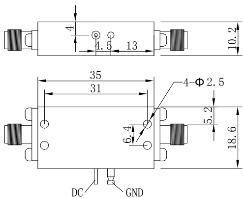
UNIT:mm XB-02A
