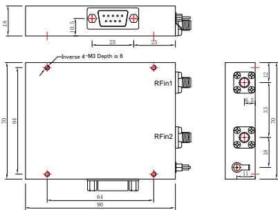
XB-17A UNIT:mm
