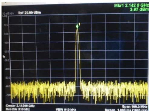
fo=2.142GHz span=100MHz Spectrum
